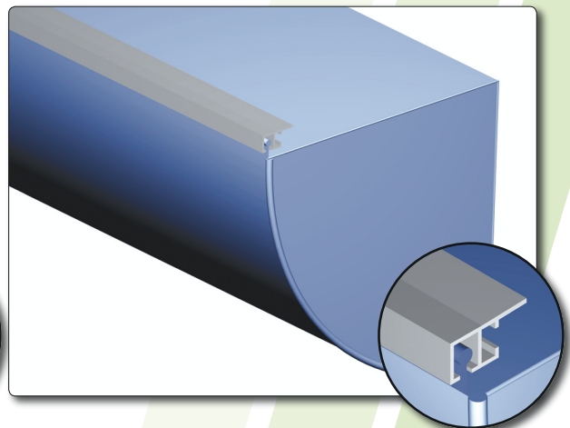
Viertel runder Auslass, mit Fasttrack in Wingrail Schiene montiert
