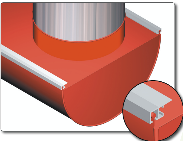
Halbrunder Auslass mit Fasttrack in Wingrail Schiene montiert
