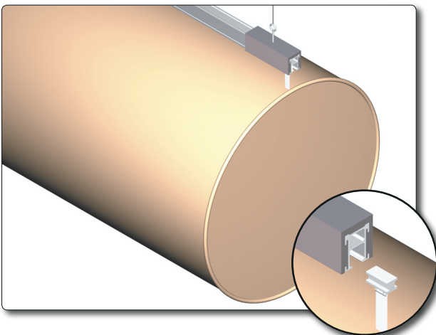
Auslass mit Gleitern, abgehängter Flexrail mit Strap-ups Abhänger
